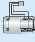
Масловоздушное смазывание
