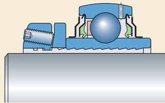
д) Фиксация SKF ConCentra, шарикоподшипниковые узлы
