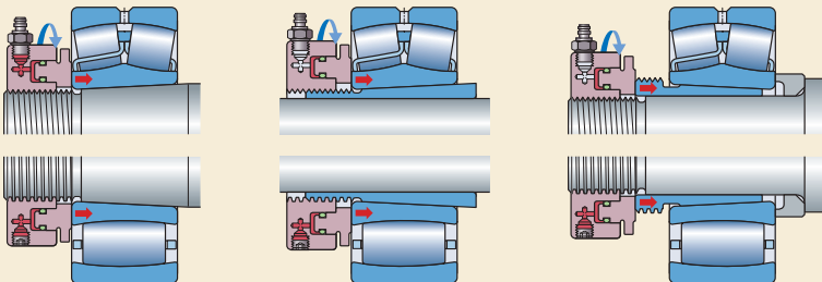
Конический вал
