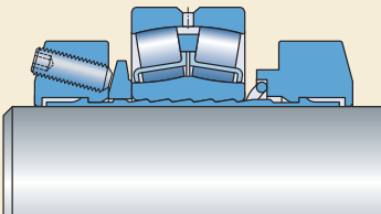
е) Фиксация SKF ConCentra, роликоподшипниковые узлы
