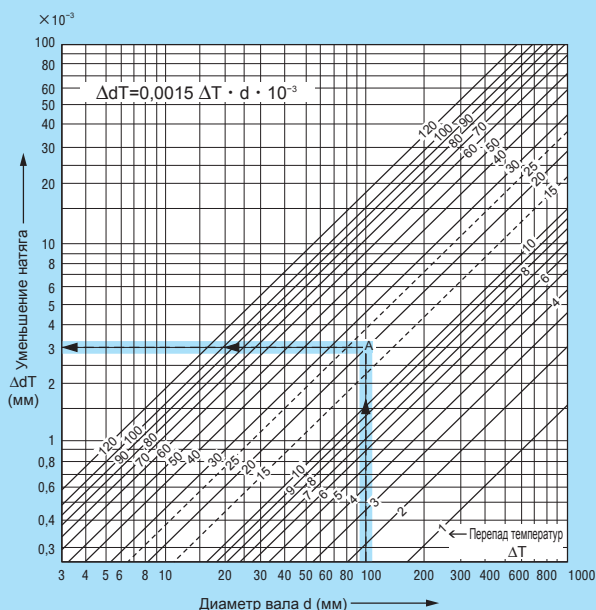
Рис. 8.2 Уменьшение натяга внутреннего кольца из-за перепада температур
