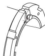
Рис. 8.16 Насадка с фиксирующим диском (Номер диаметра отверстия подшипника > 40 )
