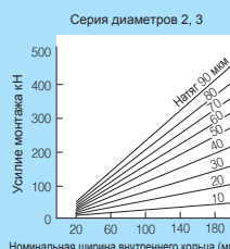
Рис. 8.48 Усилие монтажа
