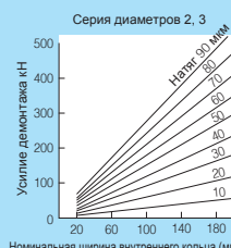
Рис. 8.46 Усилие демонтажа
