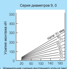
Рис. 8.49 Усилие монтажа
