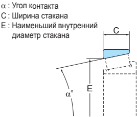
Рис. 1. Размеры субблока
