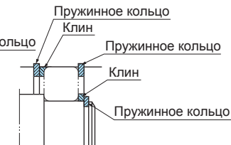
(c) Пружинное кольцо и прокладка
