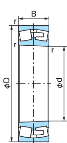
Коническое отверстие
