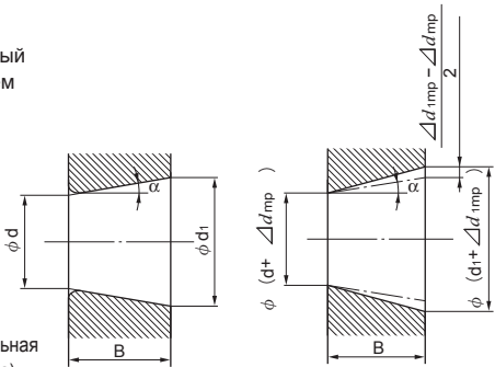
Теоретически коническое отверстие Коническое отверстие с реальными средними диаметрами при их отклонениях
