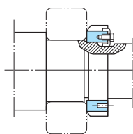
(b) Гайка вала и фиксирующий диск
