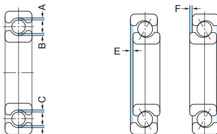
Рис 6.1 Радиальный внутренний зазор = A + B + C + D
