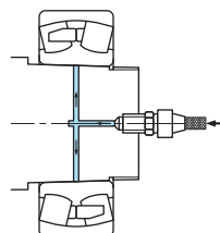
Демонтаж подшипника с помощью инжектора масла
