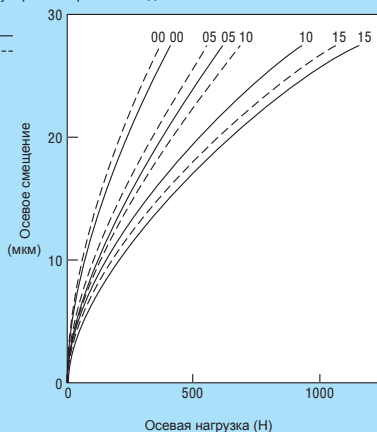
Рис. 8.4 Осевая нагрузка и осевое смещение
