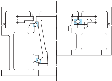
Пример монтажа конических роликовых подшипников и конического роликового подшипника с перекрещивающимися роликами
