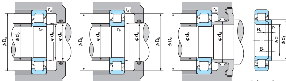
Г-образный упорный буртик
