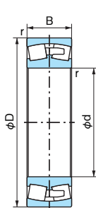
Цилиндрическое отверстие
