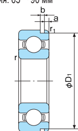
С канавкой под пружинное кольцо (N)
