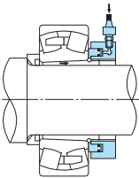
Рис. 8.45 Гидравлическая гайка
