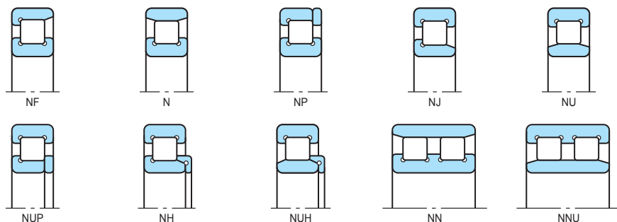
Рис. 1. Конфигурации цилиндрических роликовых подшипников
