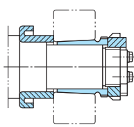
Рис. 8.17 Монтаж съемной втулки
