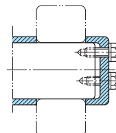
(c) Концевая пластина и болты
